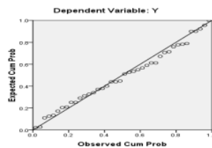
Gambar 1. Uji Normalitas
